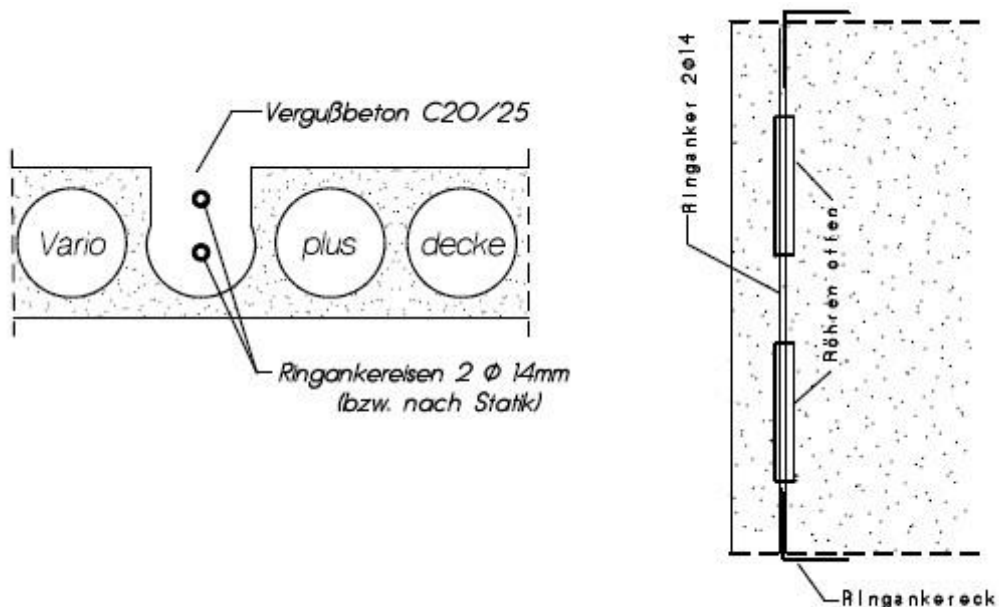
Draufsicht Schnitt
