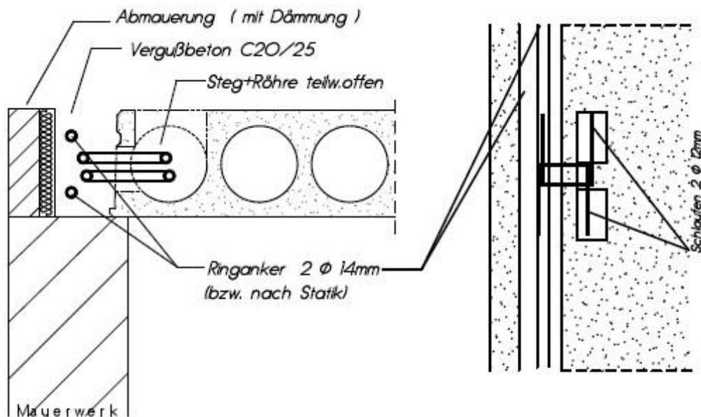
Schnitt
