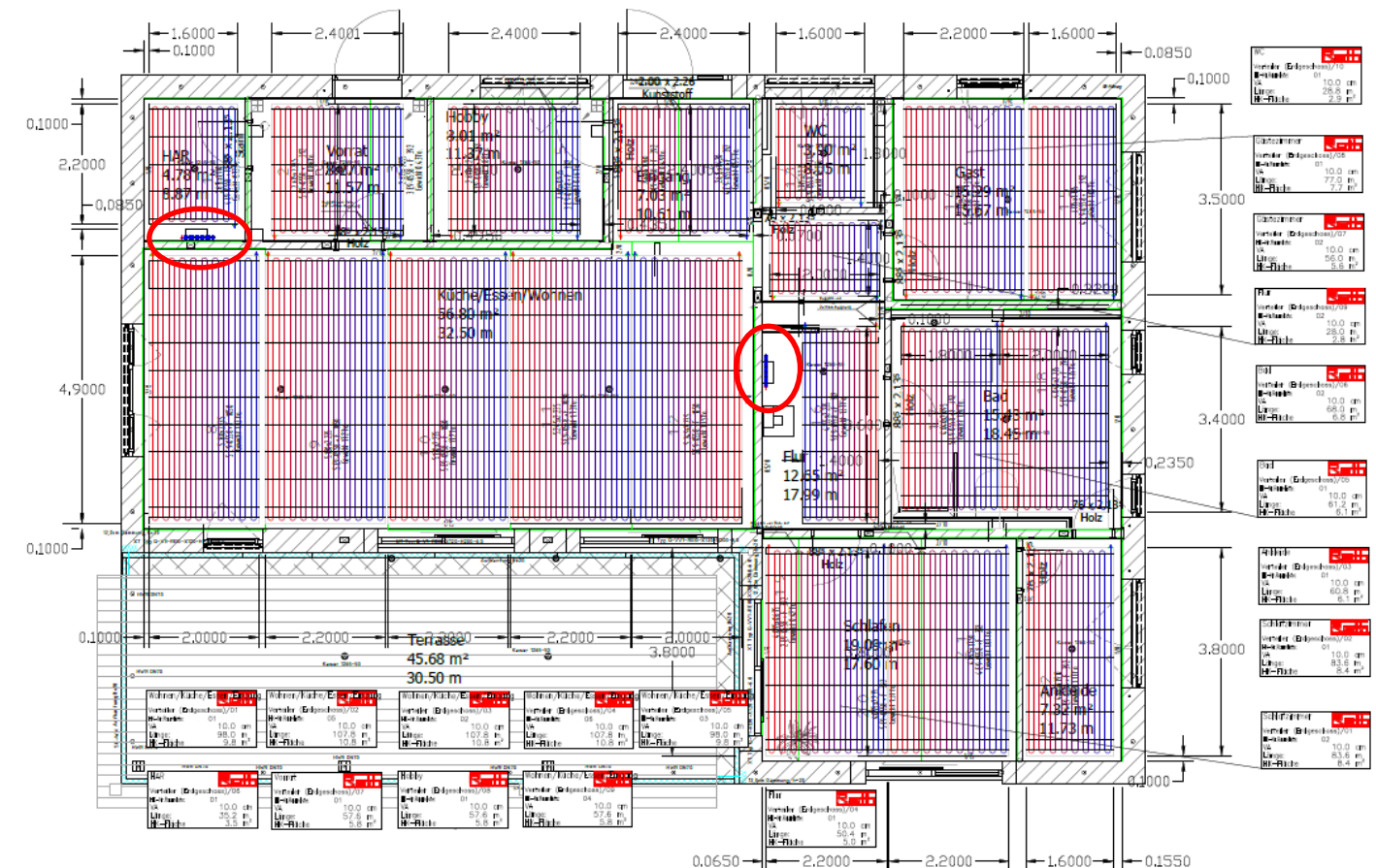
Beispielhafter Verlegeplan mit Lage Heizkreisverteiler
