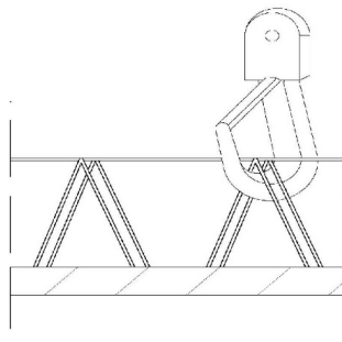
Einhängung Karabinerhaken in Gitterträger-Knotenpunkte
