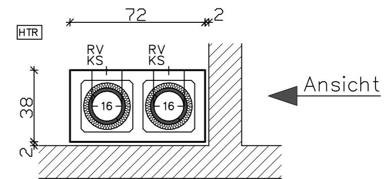
Querschnitt KG
